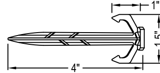
4" ECODUTY STAKE
