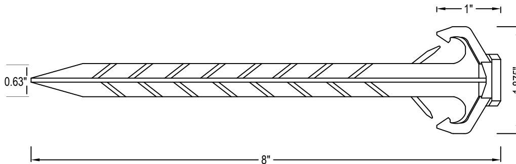
FRONT VIEW 8" 300 PCS PER CASE 70 CASES PER PALLET
